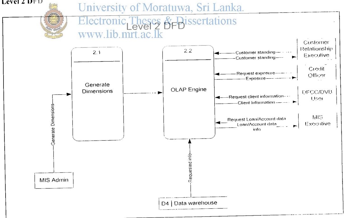
Level 2 DFD
