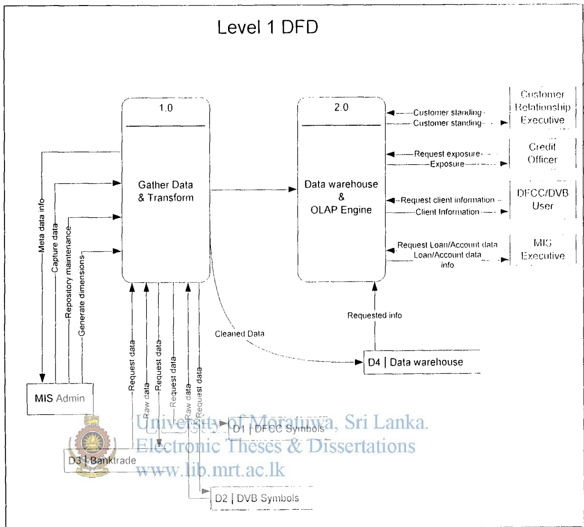
Level 1 DFD
