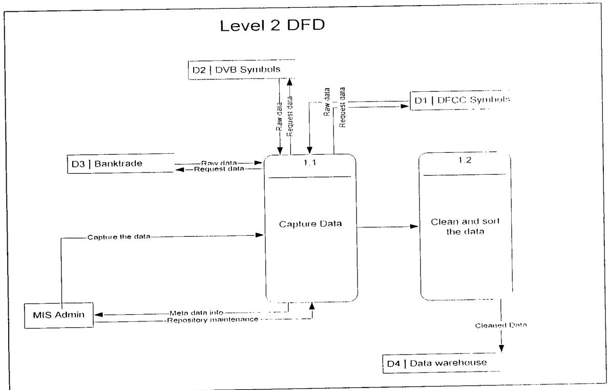
Level 2 DFD
